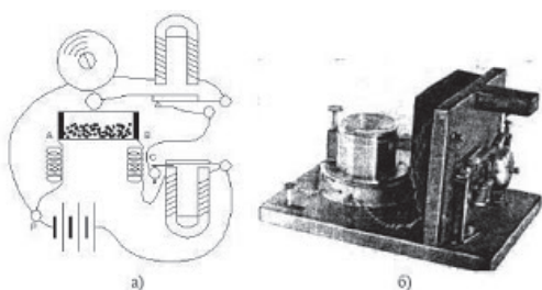
Кристалдин (фактически радиоприемник без усилительного каскада).
