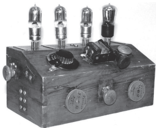
Установка демонстрирующая кристадинный эффект.
