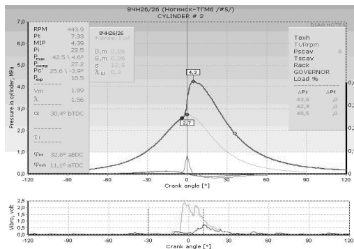
Рис. 3. Диаграмма цилиндра № 2.
