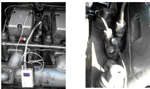
Рис. 2. Установка прибора на дизеле 3 А-6 Д49: а – датчик давления на индикаторном кране цилиндра; б – вибродатчик на корпусе форсунки.
