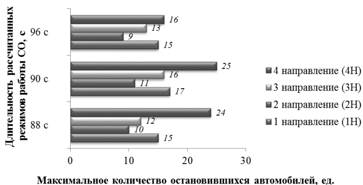
Рис. 3. Гистограмма зависимости количества остановившихся автомобилей от длительности полученных режимов работы.
