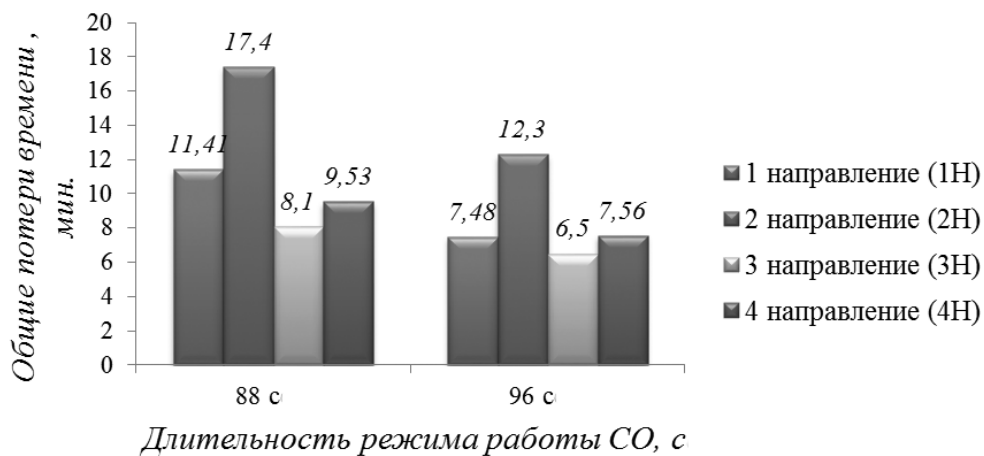
Рис. 5. Гистограмма изменения общих потерь времени при существующем и внедряемом режимах работы светофорных объектов.
