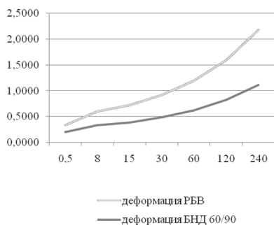
Рис. 2. График деформаций РБВ и исходного битума при температуре -28^{\circ}\text{C} .
