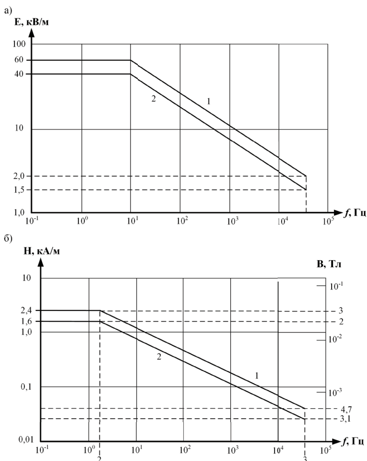
Рис. 2. Предельно-допустимые значения напряжённости E электростатического поля (а) и параметров H и B магнитного поля (б) согласно международным стандартам: 1 – пиковые значения; 2 – эффективные значения.
