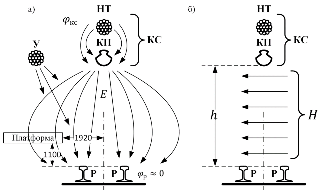
Рис. 1. Электрическое поле в зоне контактной сети (а – электростатическое поле; б – электромагнитное поле).
