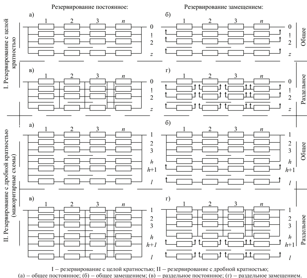
Рис. 2. Сочетания способов структурного резервирования.
